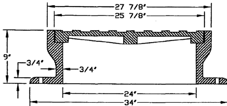
SECTION -XX
