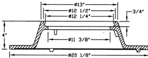
BODY SECTION -XX
